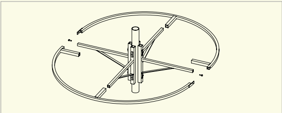
PIX02 / PIX03 Potence circulaire pour composer vos décorations 3D Diamètre intérieur : réglable
