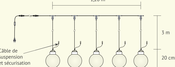
Câble de suspension et sécurisation de 60 cm
